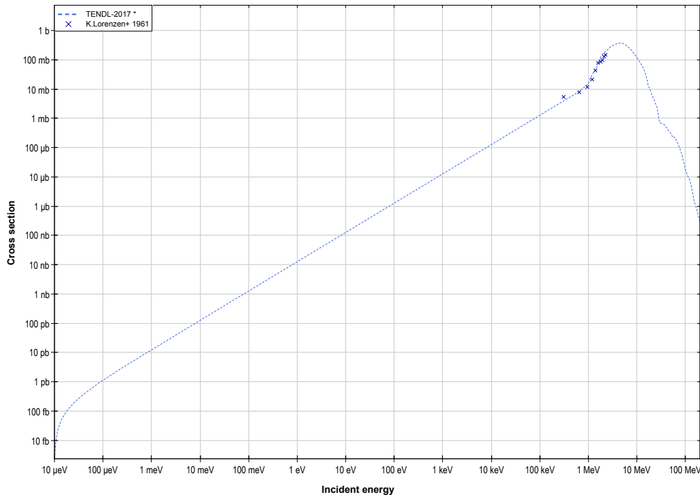
O16 (t,n) or F18 production log-log
