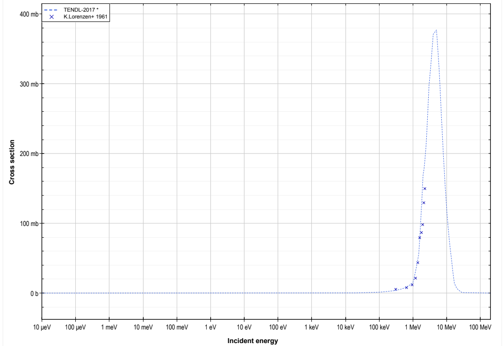
O16 (t,n) or F18 production lin-log
