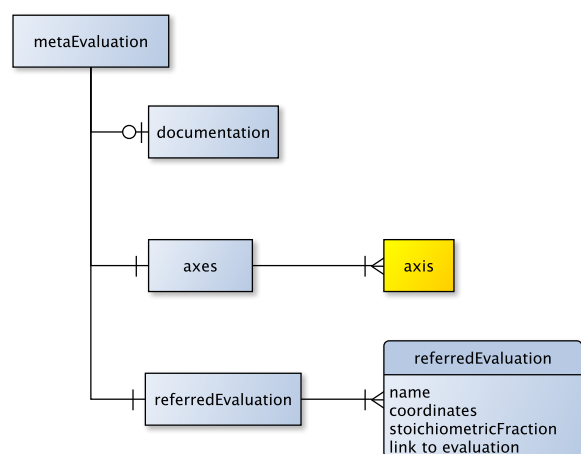
FIG. 24 The <metaTargElement> element.
