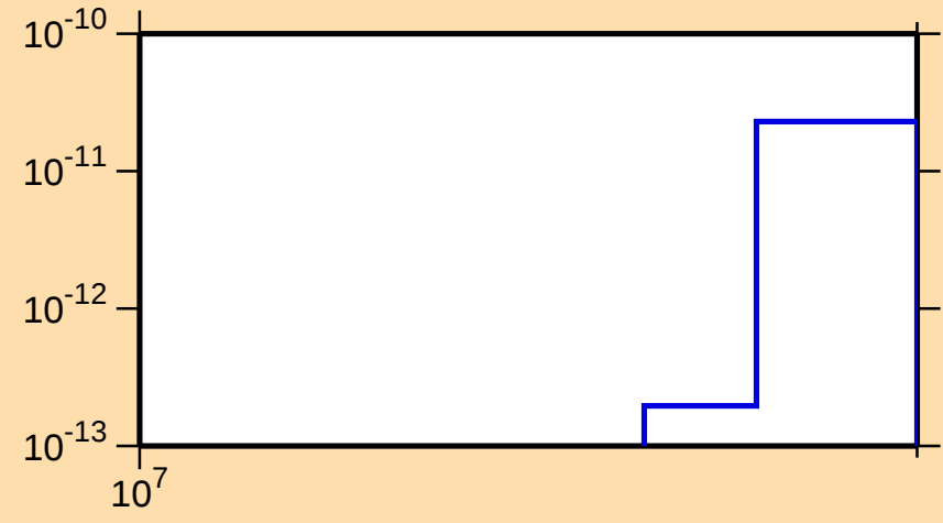
\sigma vs. E for ^{186}\text{Os}(\text{mt } 45)
