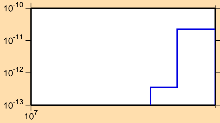
\sigma vs. E for ^{185}\text{Os} (mt 45)
