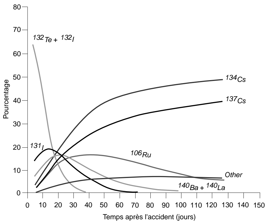
Figure 8. Débit de dose absorbée dans l'air dans une zone contaminée de la Fédération de Russie au cours des tout premiers mois suivant l'accident de Tchernobyl : Part revenant aux différents radionucléides
