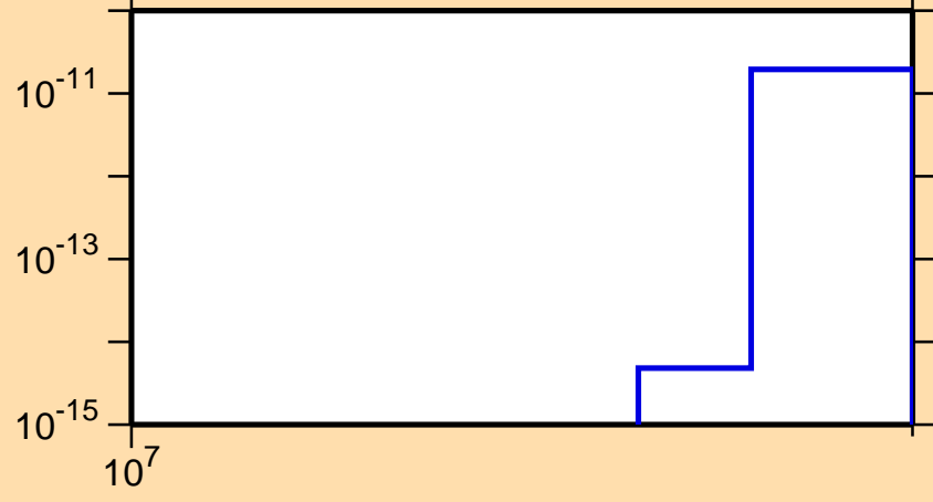
\sigma vs. E for ^{126}\text{Xe}(\text{mt } 45)
