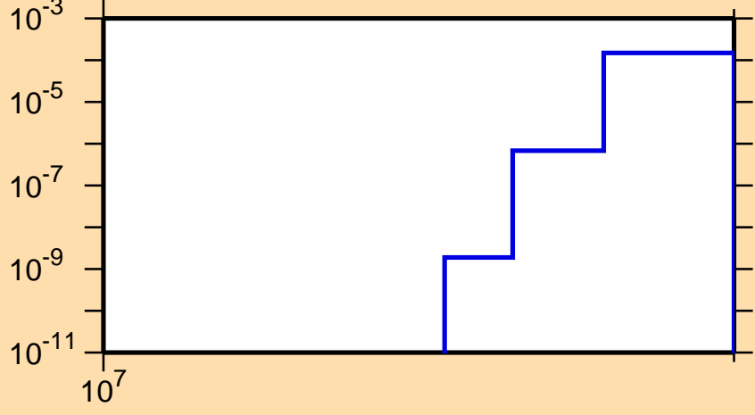
\sigma vs. E for ^{67}\text{Ga} (mt 45)
